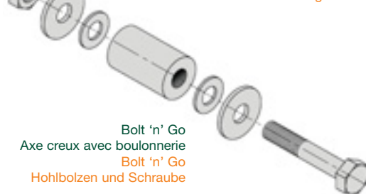
Axe plein et circlips Flachbolzen mit zwei Schließringen
